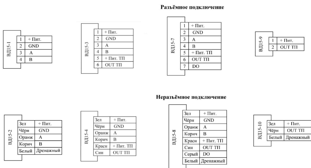
Рисунок 1. Варианты исполнения и подключения датчика ВД15
