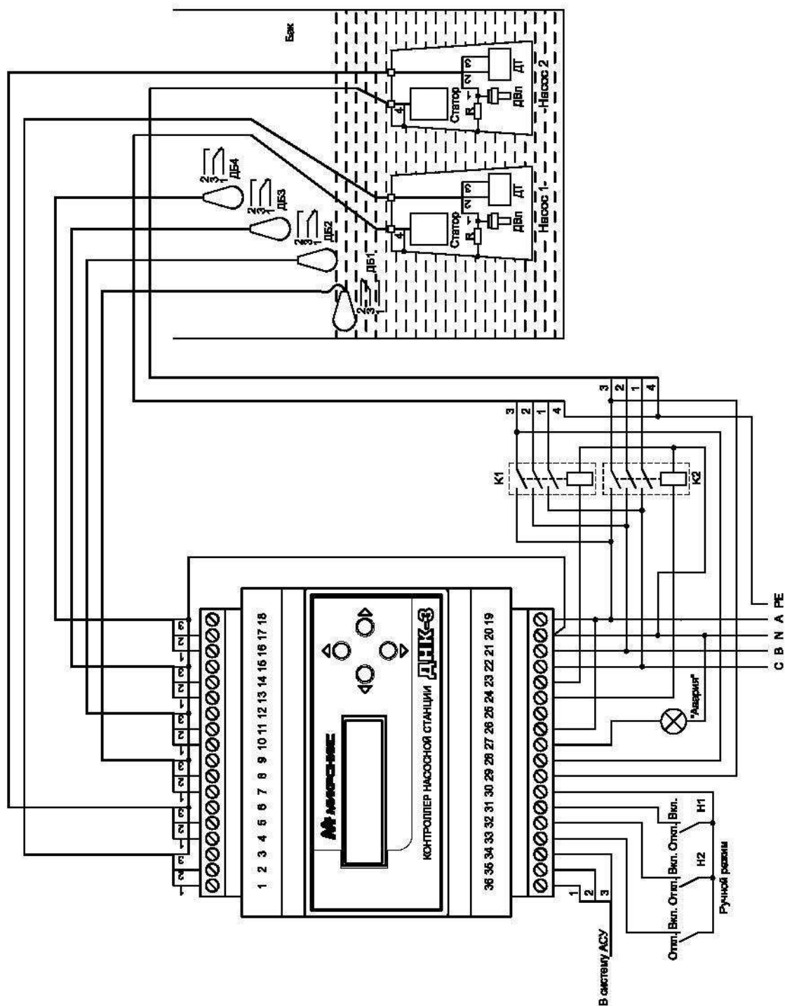
Рисунок 16 - Рекомендуемая схема включения
