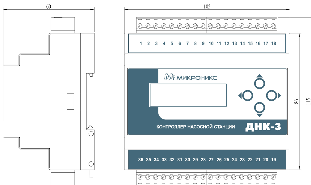
Рисунок 1б - Габаритные размеры изделия
