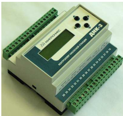
Рисунок 1а - Внешний вид устройства
